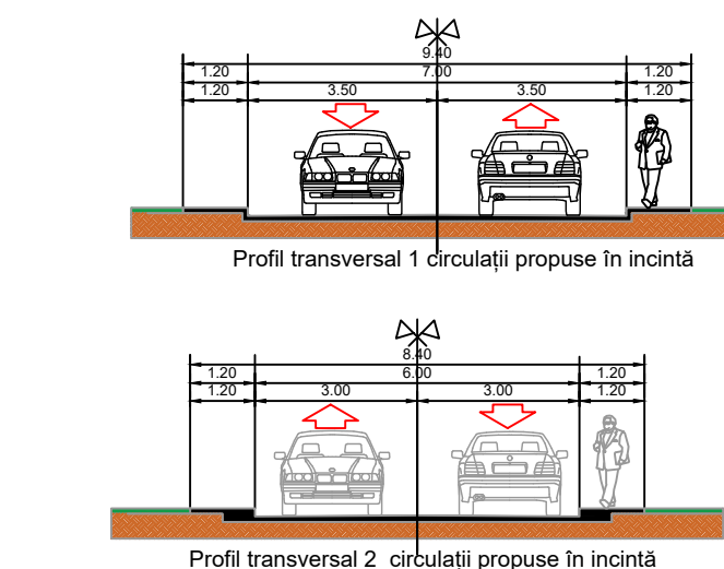
PROFILUL TRANSVERSALE CIRCULAȚIILOR PROPUSE ÎN INCINTĂ
